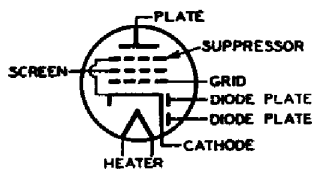
DUPLEX-DIODE PENTODE
