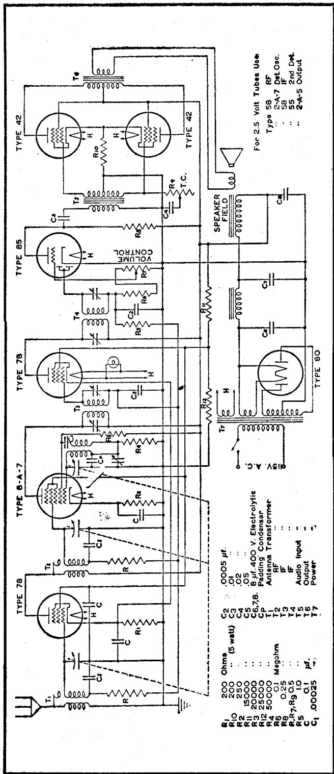
RECEPTEUR A 7 TUBES SUR SECTEUR ALTERNATIF
