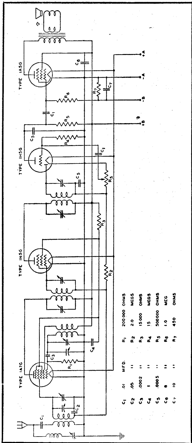
RECEPTEUR BATTERIE 1.4 VOLT AVEC A. V. C.
