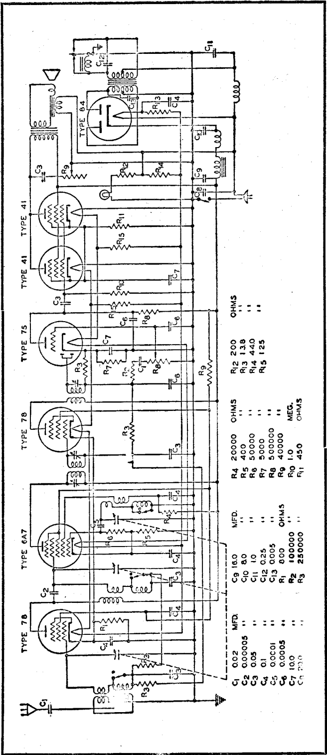
RECEPTEUR 32 VOLTS. A 7 TUBES. POUR FERME
