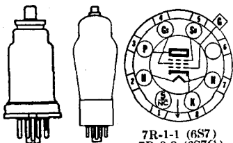
7R-1-1 (6S7) 7R-0-8 (6S7G)
